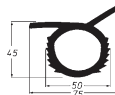
S 45/50/75 Eck (für 30er - 40er Fugen) (do fug 30-40 mm)
