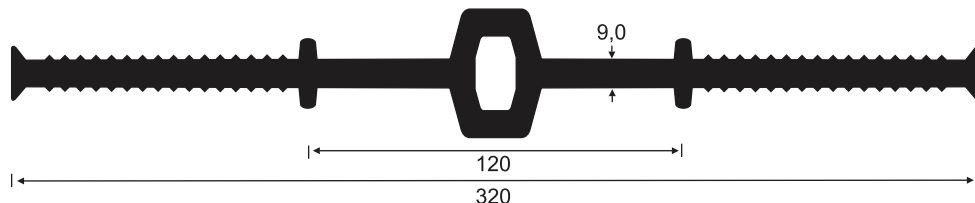
Taśmy dylatacyjne, wewnętrzne, ze zbrojeniem sprężonym i pętlami mocującymi, czarne, DIN 18541
