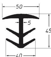
EP 45/50/40 (für 30er Fugen) (do fug 30 mm)
