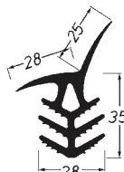
EP 35/28/28 Eck (für 20er Fugen) (do fug 20 mm)
