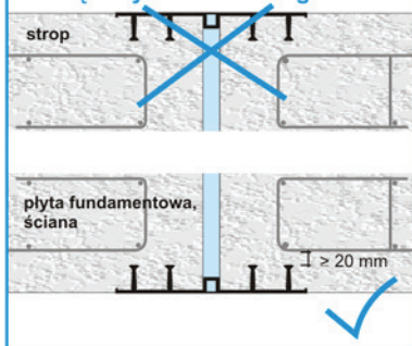
montaż zewnętrznych taśm do fug
