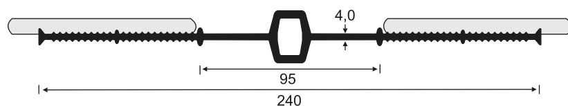
Taśmy dylatacyjne, wewnętrzne, ze zbrojeniem sprężonym i pętlami mocującymi, czarne, DIN 18541
