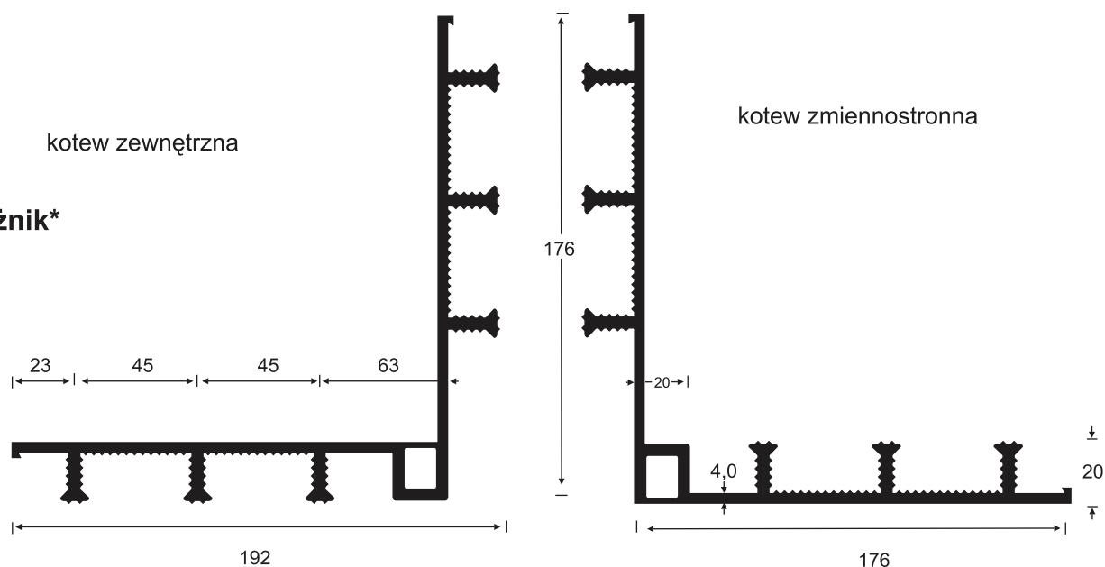
Taśmy dylatacyjne, zewnętrzne, czarne, norma zakładowa
